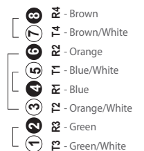
TIA (T568A)
